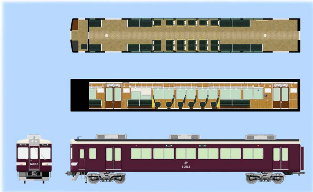
6300系（先頭車）リニューアル外観、内装イメージパース
