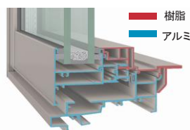
アルミ樹脂複合サッシ (概念図)
